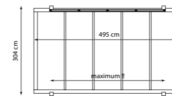
4 wand-elementen + 3 palen
