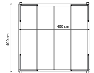
8 wand-elementen + 8 palen
