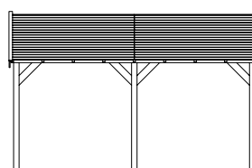
vooraanzicht
